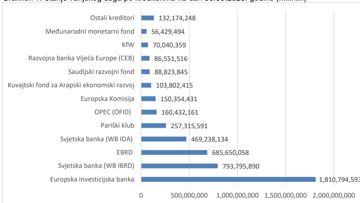
Grafikon 1. Stanje vanjskog duga po kreditorima na dan 30.09.2025. godine (mil.KM)
